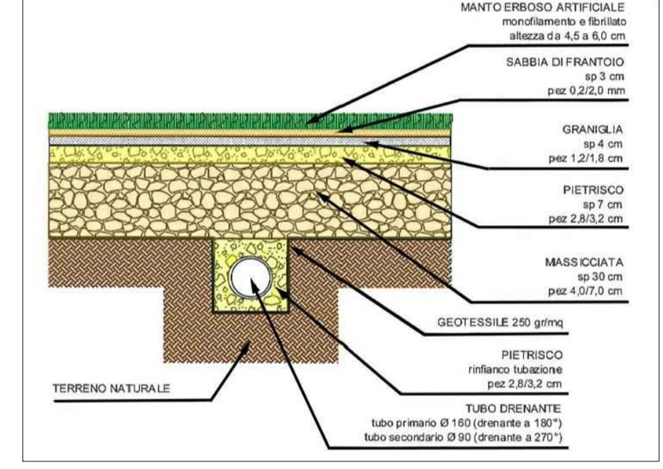
SEZIONE 1:20
