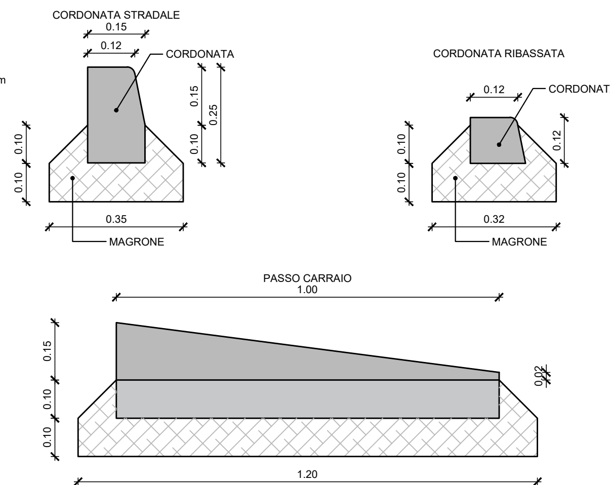
PARTICOLARE CORDONATA C1 (cordinata stradale) scala 1:10
