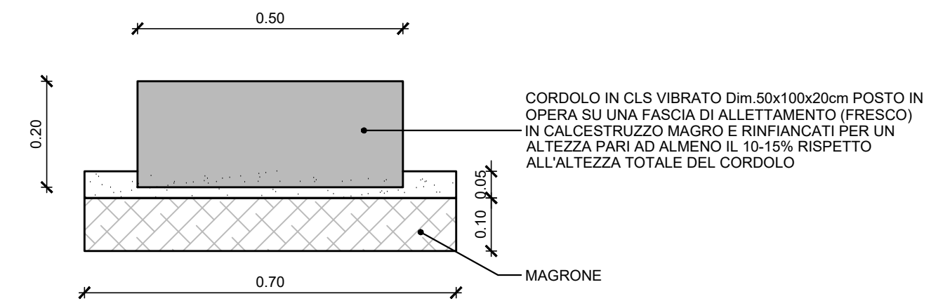
PARTICOLARE CORDONATA C2 (separatore per pista ciclabile) scala 1:10
