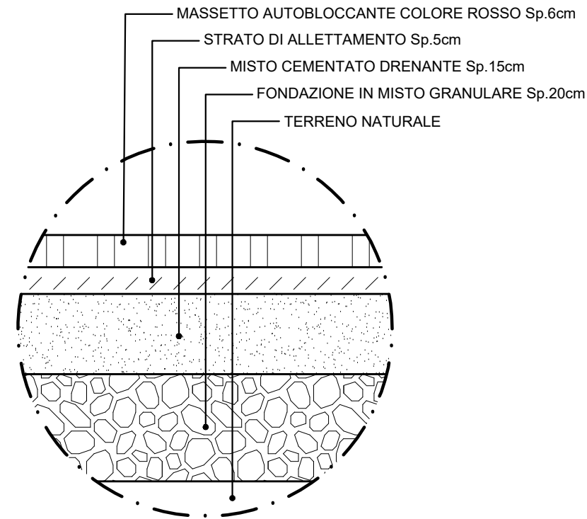
PARTICOLARE PAVIMENTAZIONE P4 (marciapiede pavimento autobloccante) scala 1:10
