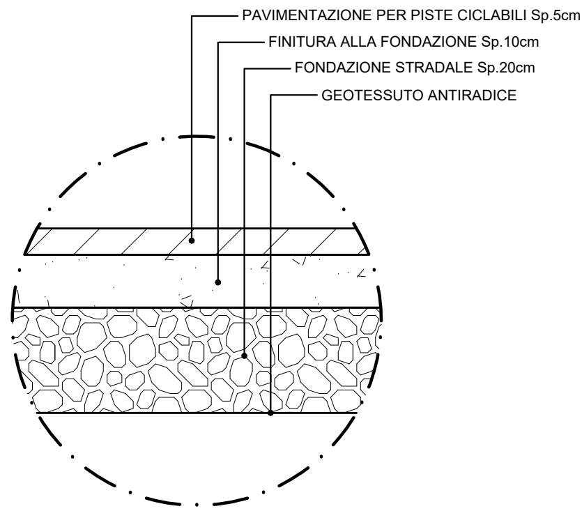
PARTICOLARE PAVIMENTAZIONE P1 (asfalto) scala 1:10
