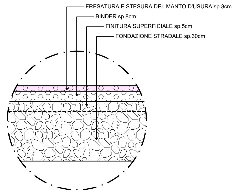
PARTICOLARE PAVIMENTAZIONE P2 (allargamento strada) scala 1:10
