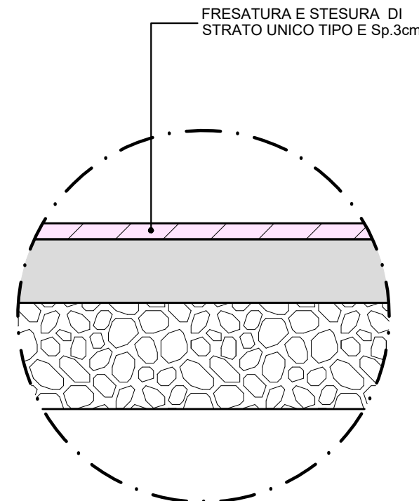
PARTICOLARE PAVIMENTAZIONE P5 (sistemazione marciapiede esistente) scala 1:10
