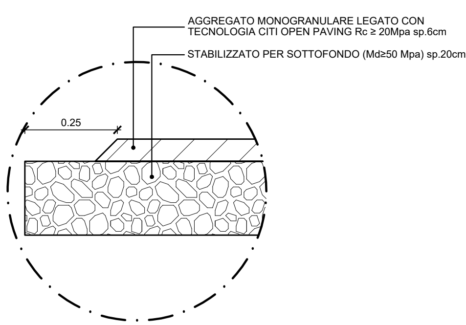
PARTICOLARE PAVIMENTAZIONE P6 (pavimentazione drenante ciclopedonale) scala 1:10
