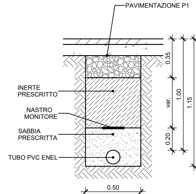
SEZIONE TIPO SCAVO (interramento linea ENEL MT) scala 1:20
