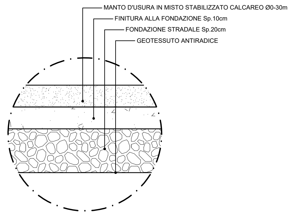
PARTICOLARE PAVIMENTAZIONE P7 (strada bianca) scala 1:10
