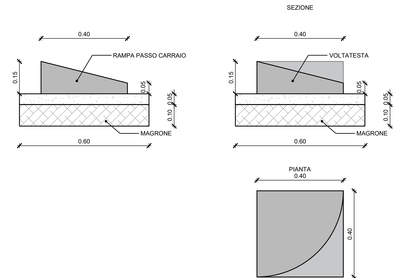
PARTICOLARE CORDONATA C3 (passo carraio e voltatesta) scala 1:10
