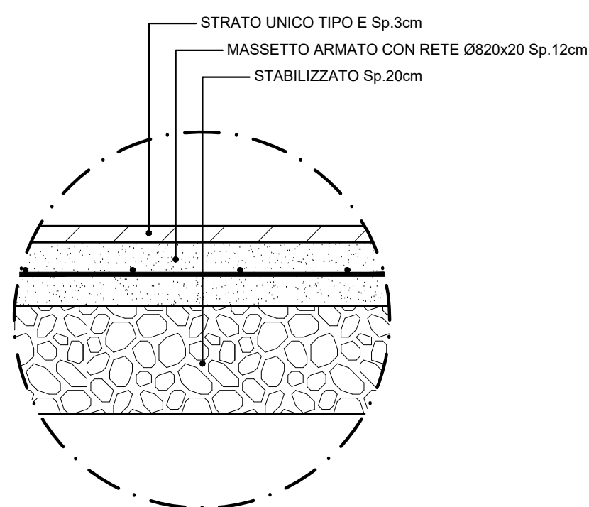
PARTICOLARE PAVIMENTAZIONE P3 (nuovo marciapiede) scala 1:10
