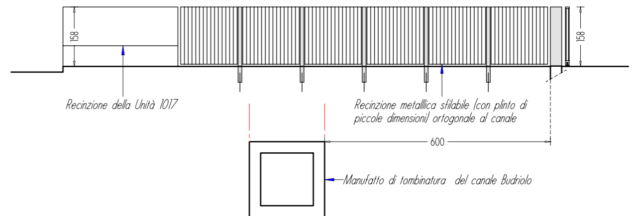
SEZIONE B-B
