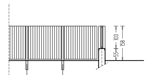
SEZIONE C-C
