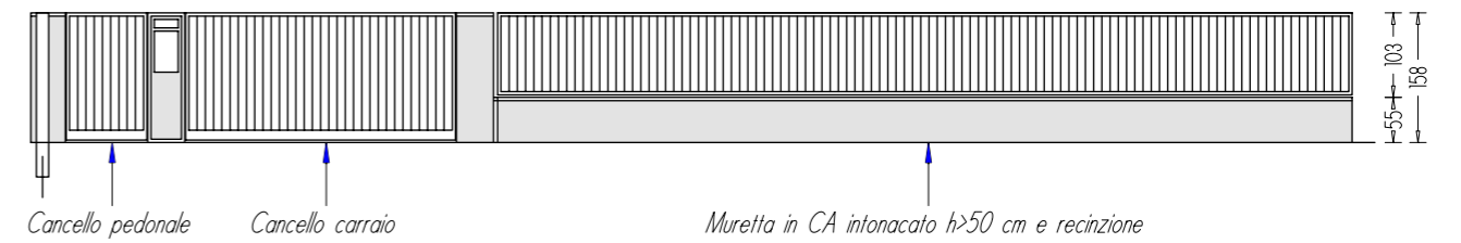
SEZIONE A-A
