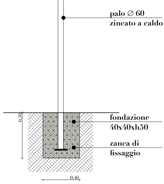
A PARTICOLARE SEGNALETICA SCALA 1:20
