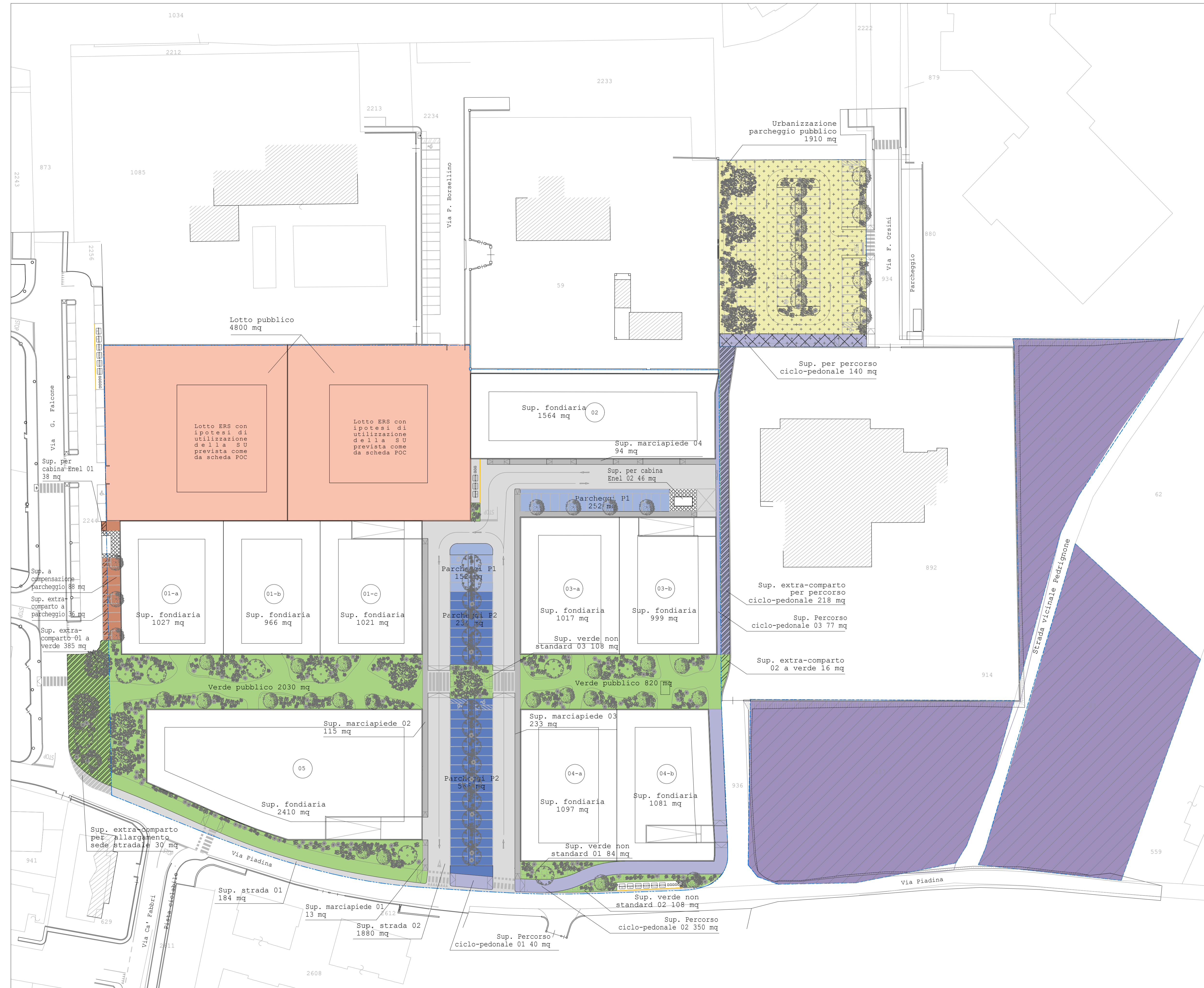
Planimetria generale di progetto con individuazione delle aree e delle opere pubbliche da cedere - Scala 1:500
