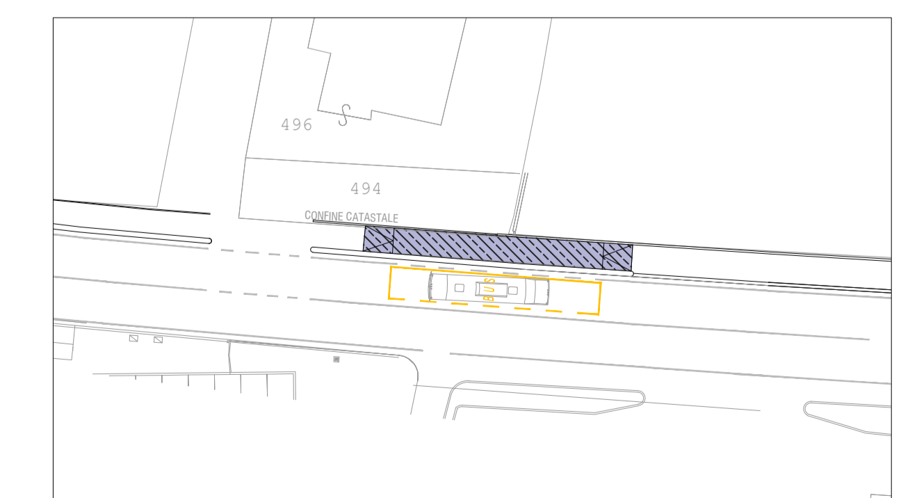
Planimetria nuova fermata autobus lungo la Via Emilia - Scala 1:500
