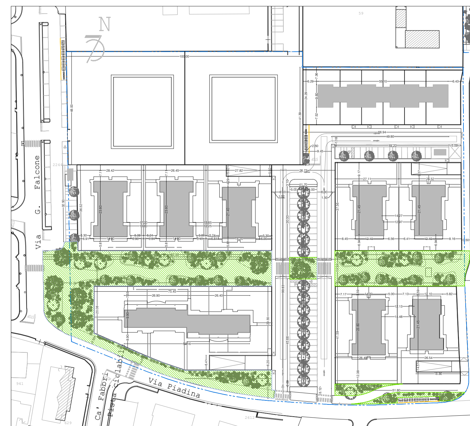
Individuazione intervento 1:1000
