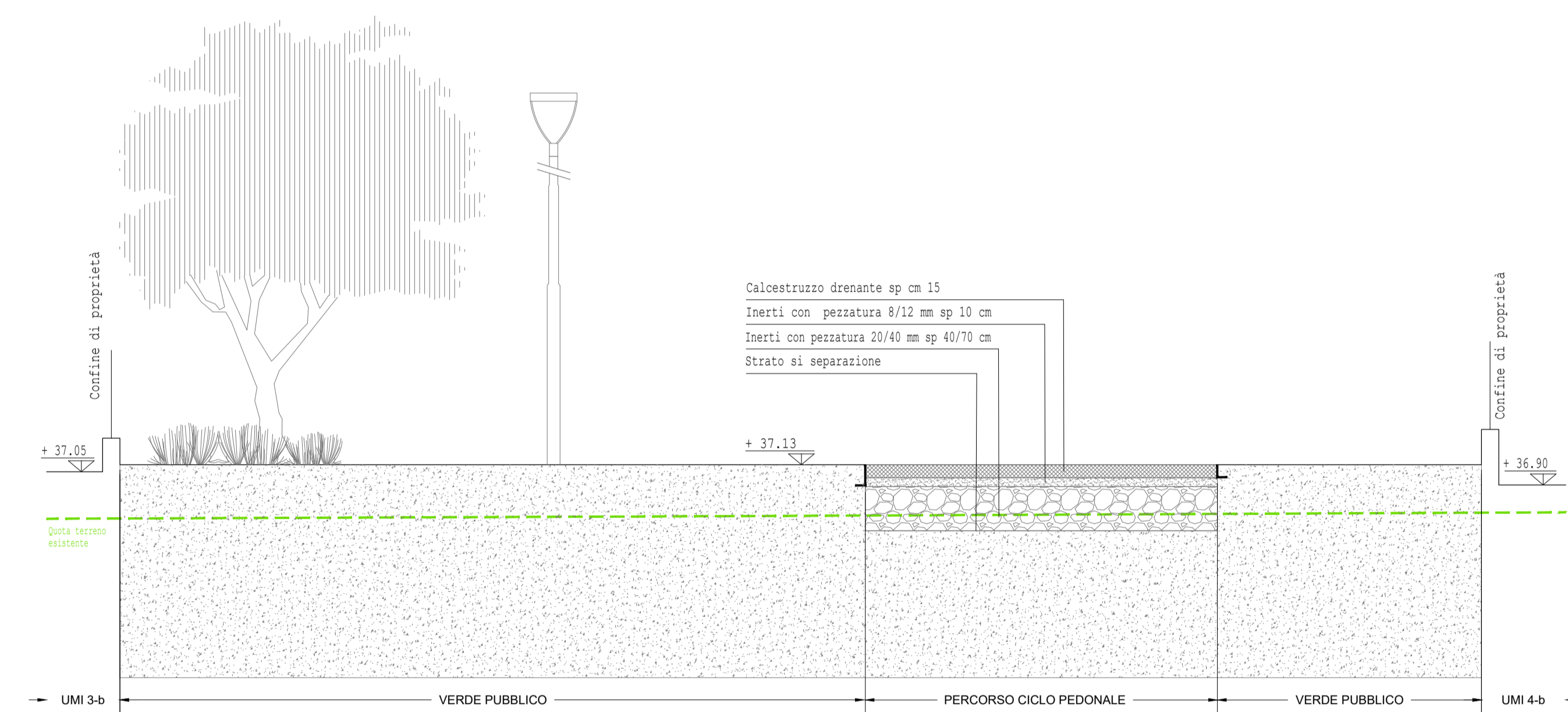
Sezione CC' 1:50
