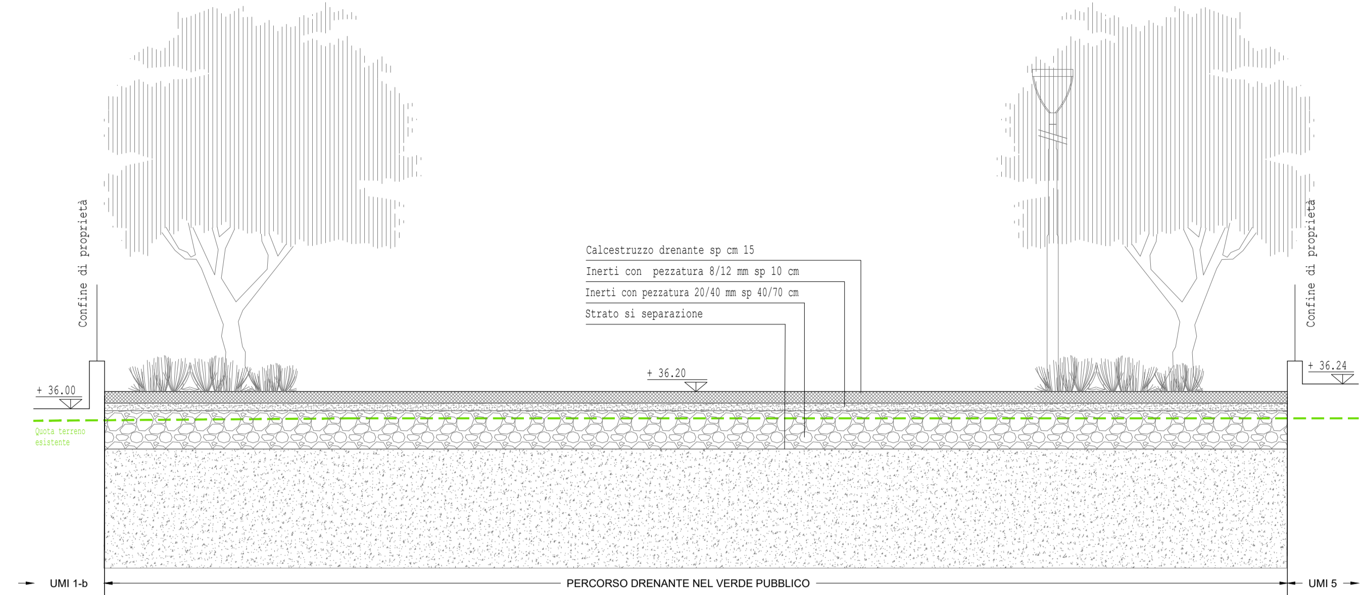
Sezione BB' 1:50
