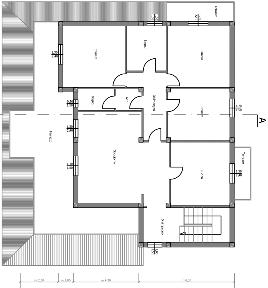
PIANO PRIMO
