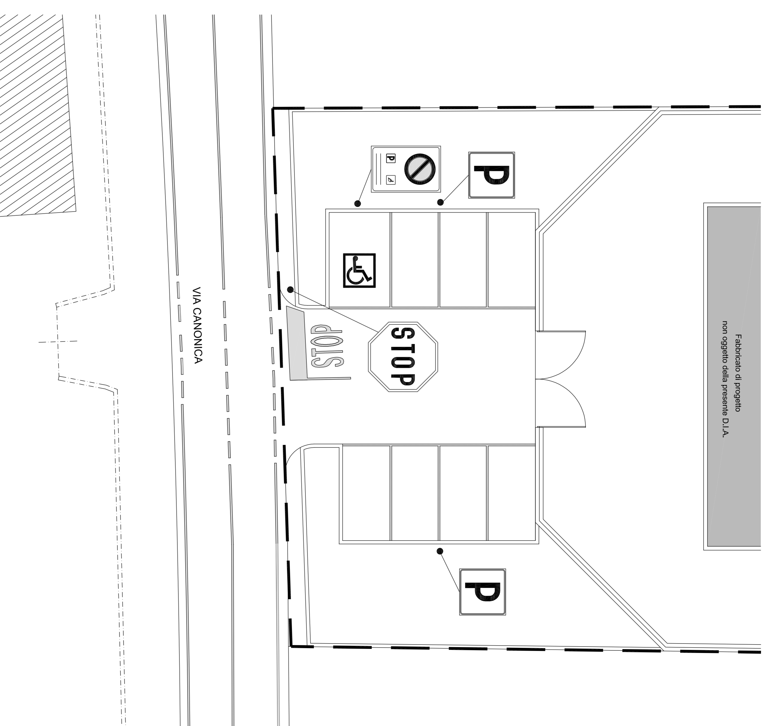
PARTICOLARE PAVIMENTAZIONE STRADE E PARCHEGGIO
